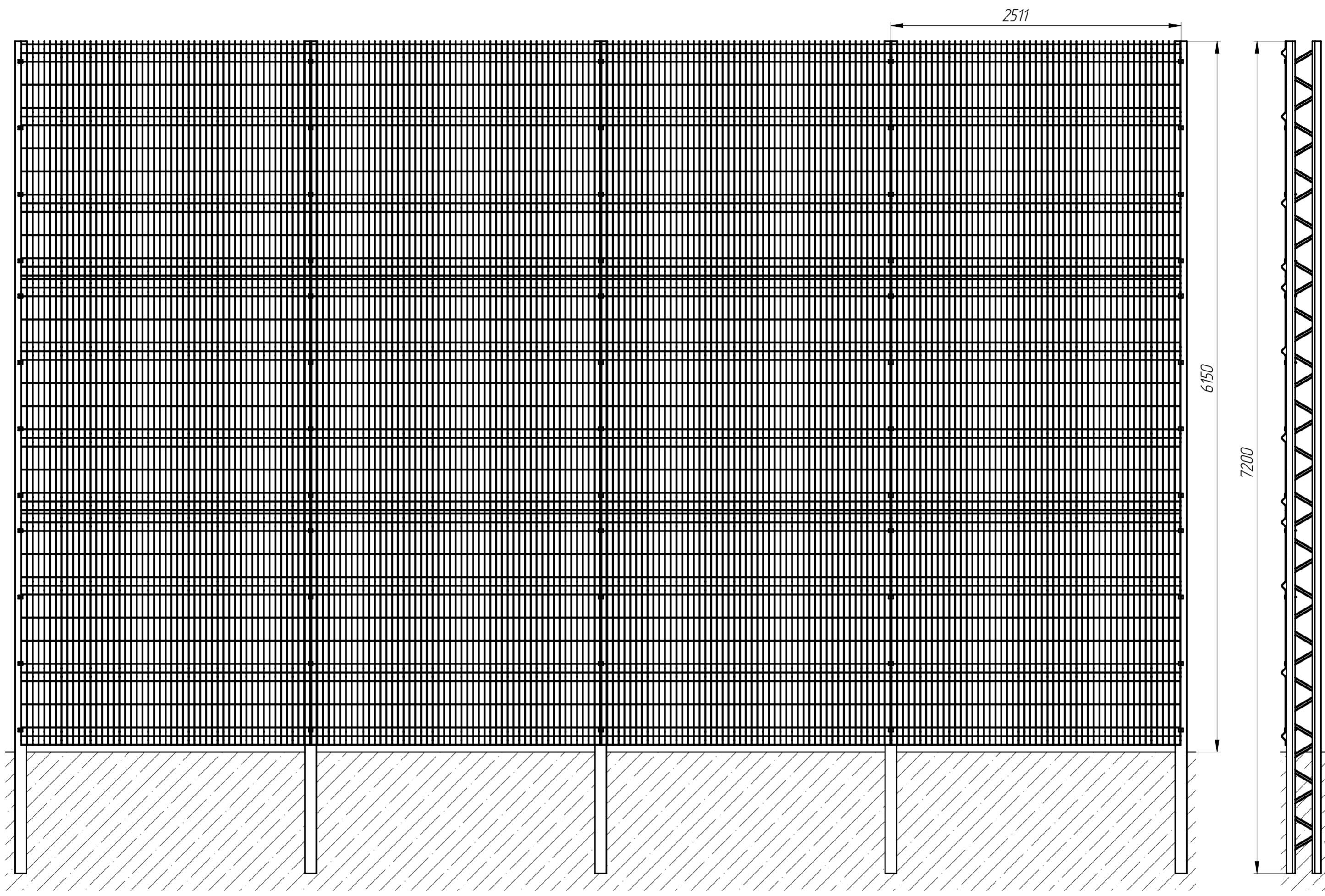
Панель оцинк. "РБ-3Д/5", (ВxШ) 2030x2500мм
